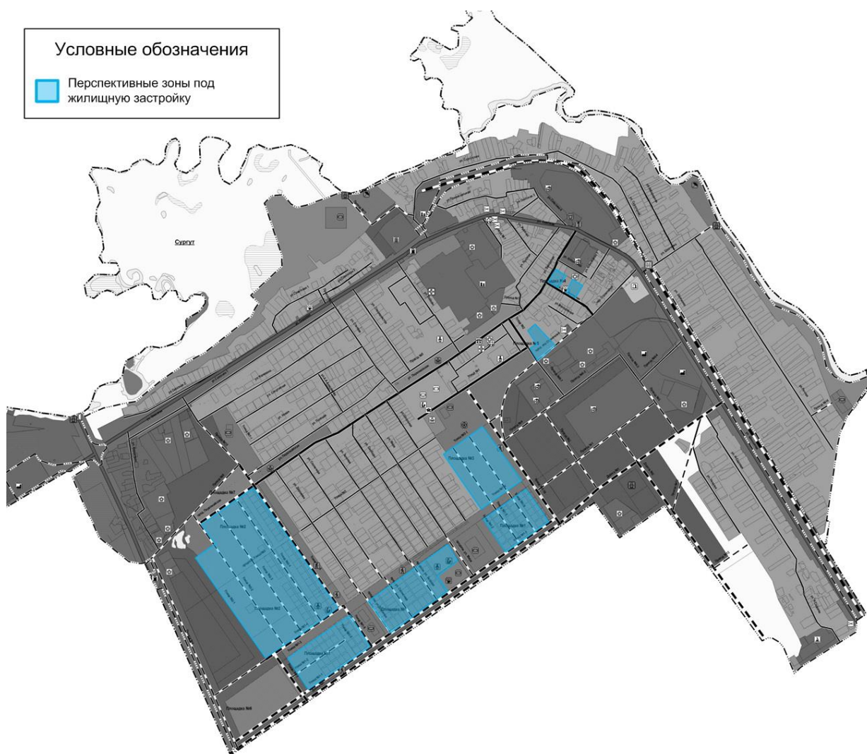
Рисунок 2.5.1 – Перспективные зоны индивидуального теплоснабжения п. Сургут
